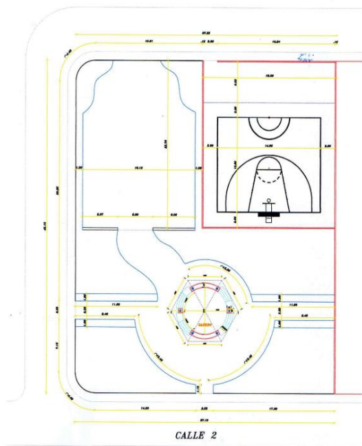
PLANTA DIMENSIONADA
