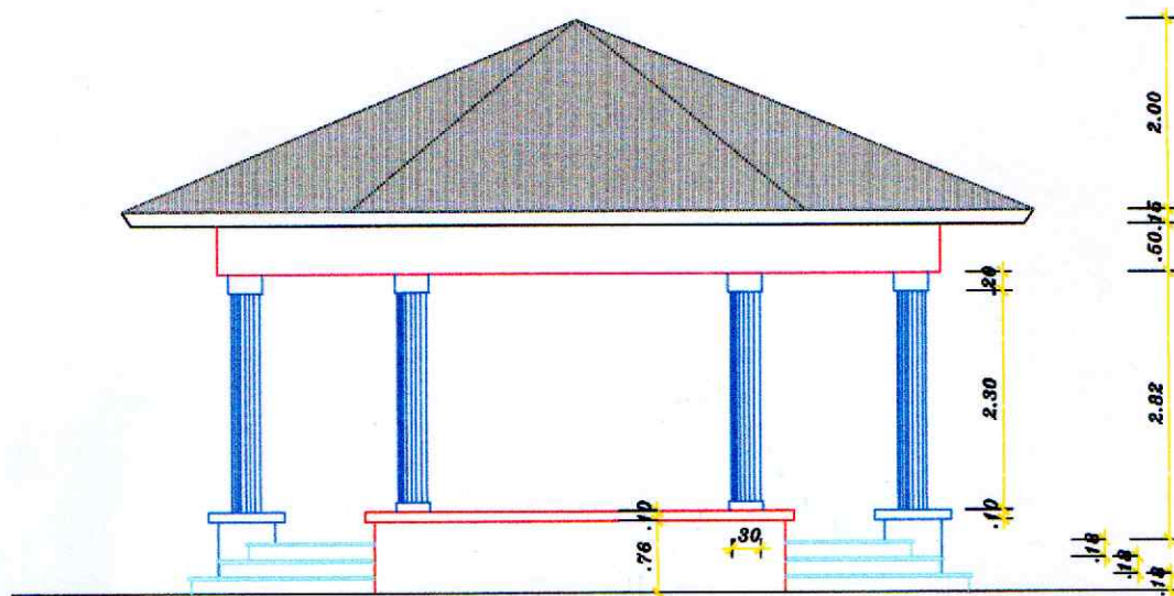
ELEVACION FRONTAL GAZEBO
